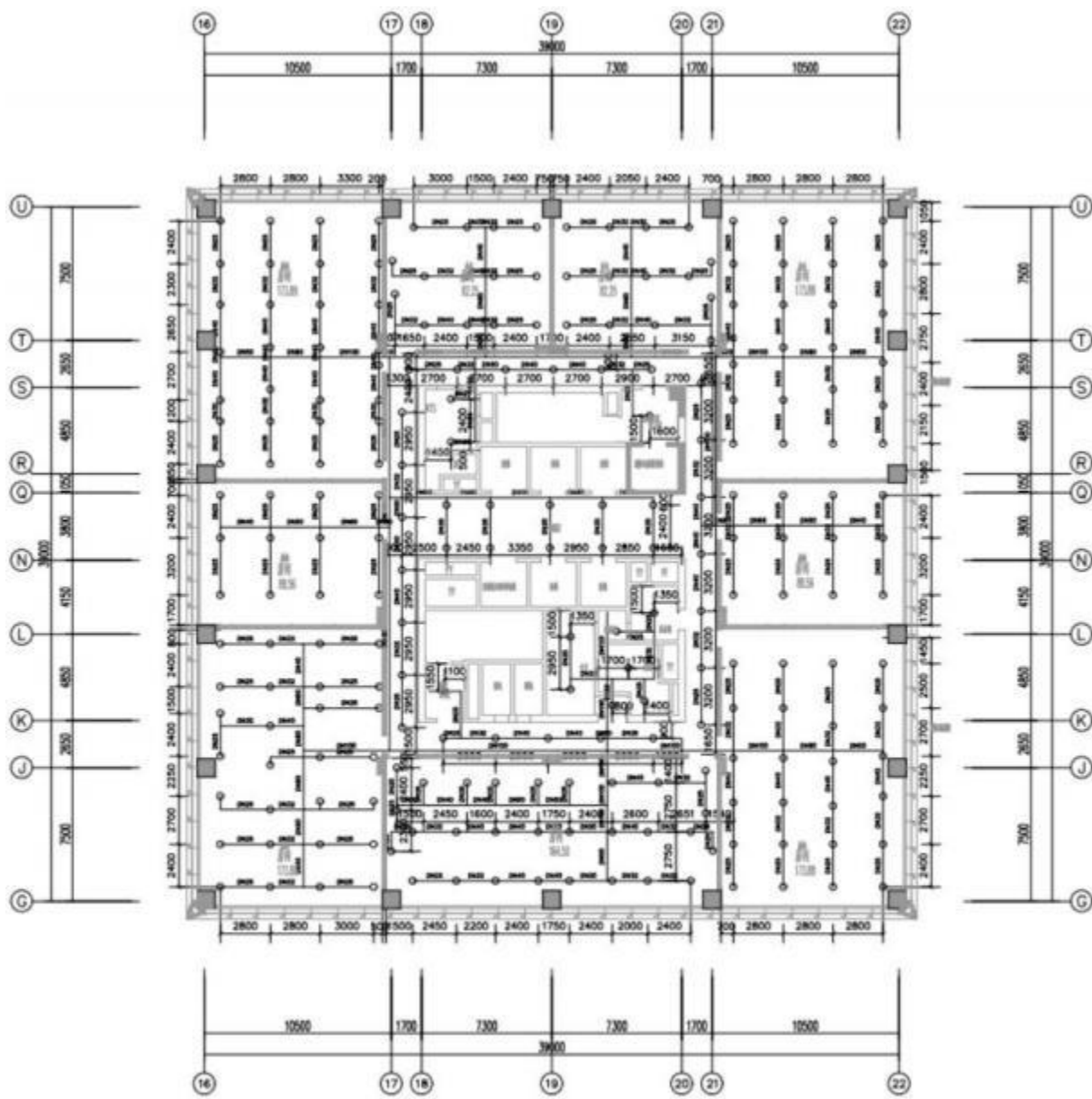
喷淋平面图 1:150
