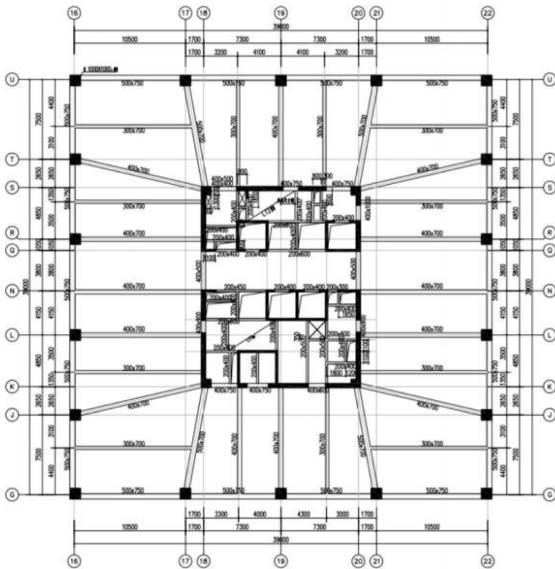
结构平面图 1:150
