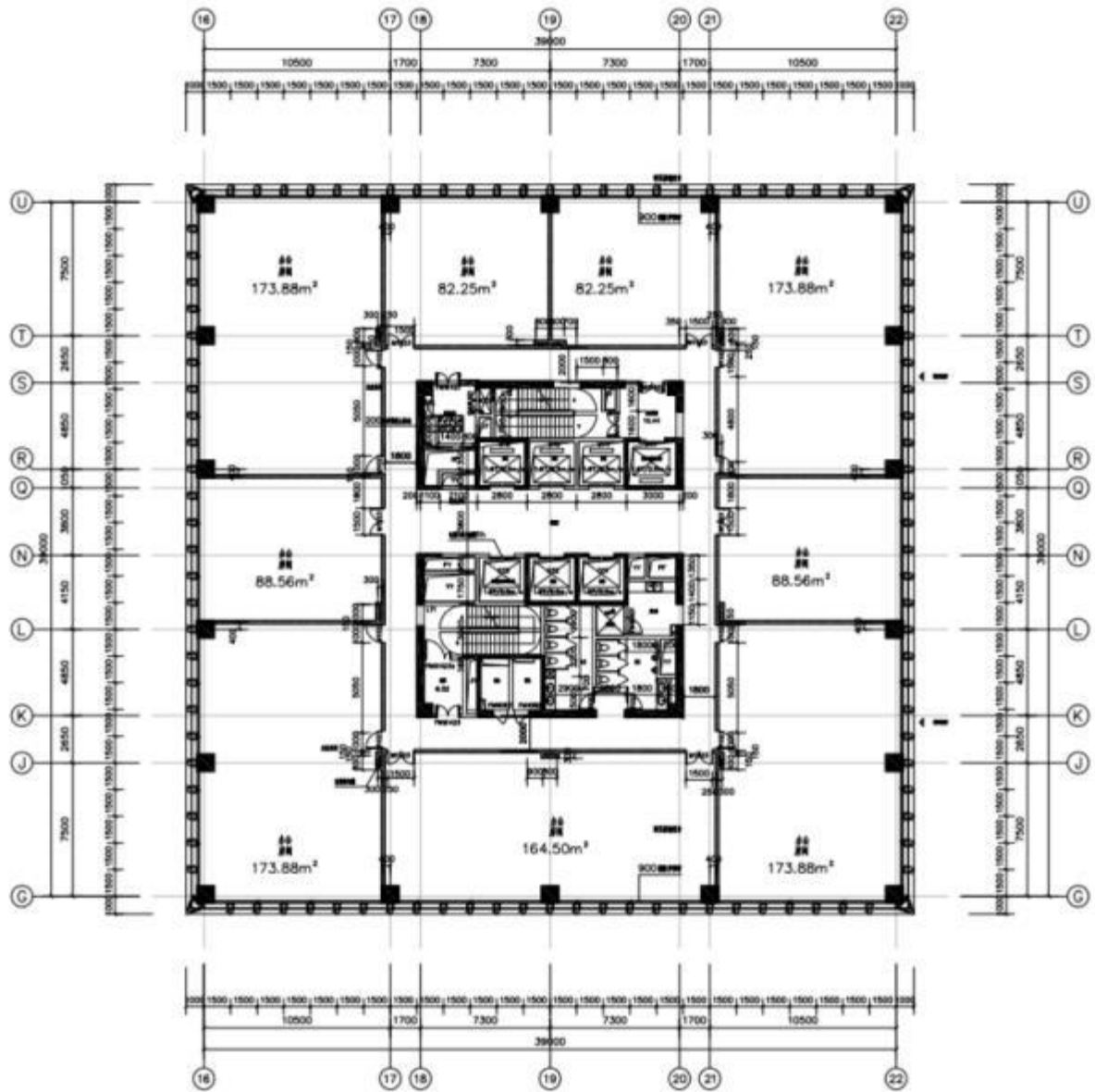
建筑平面图 1:150
