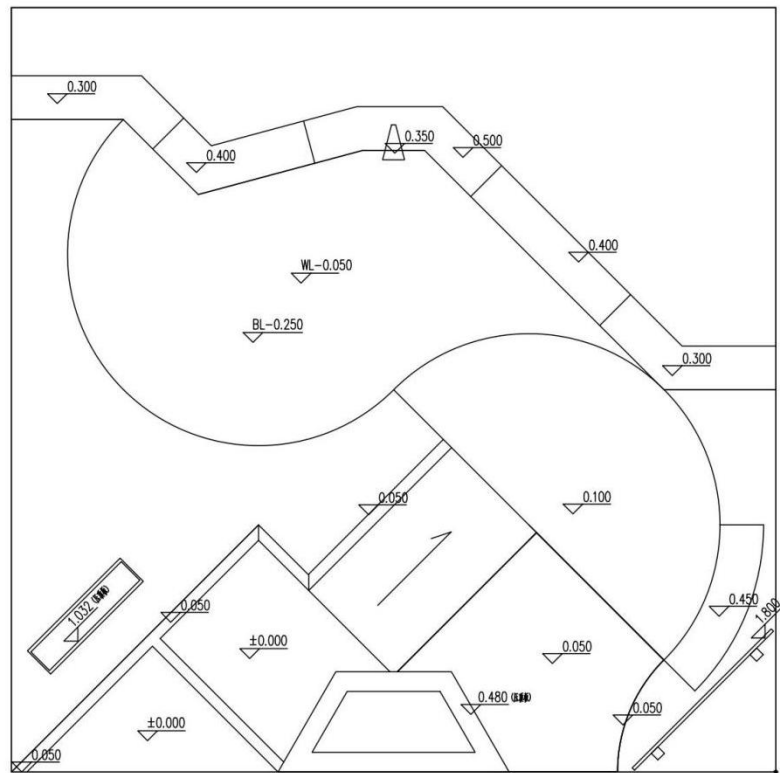
竖向标高图
