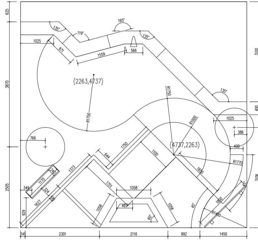
尺寸定位图
