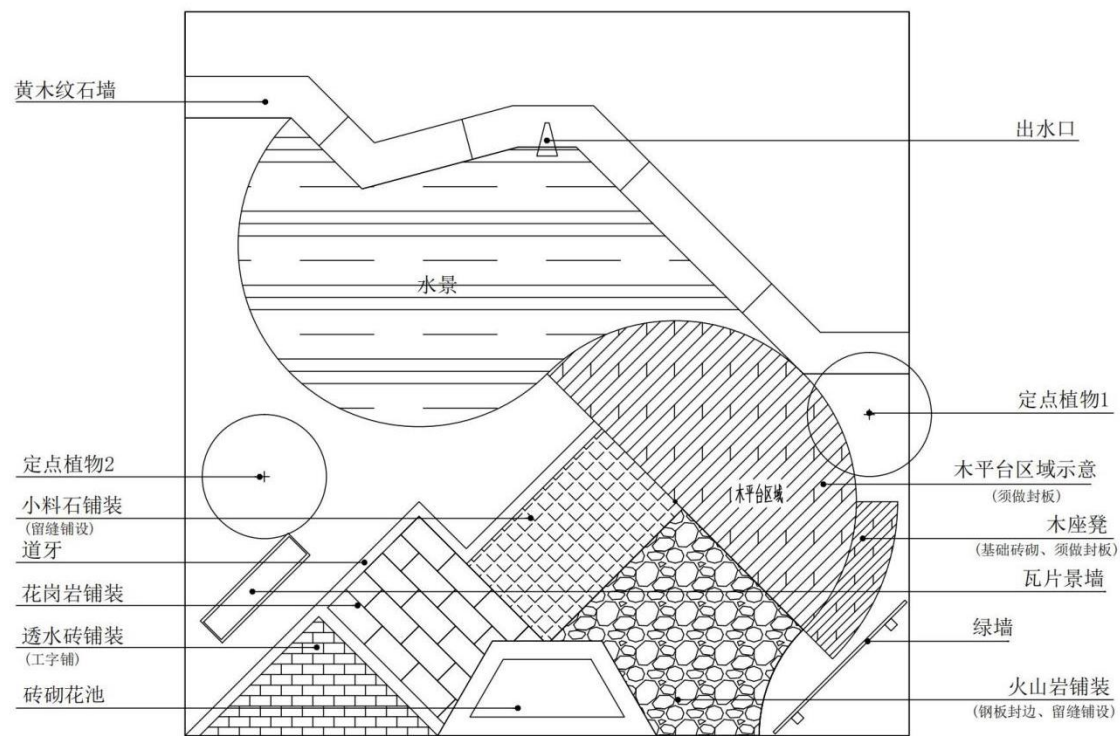
总平面图
