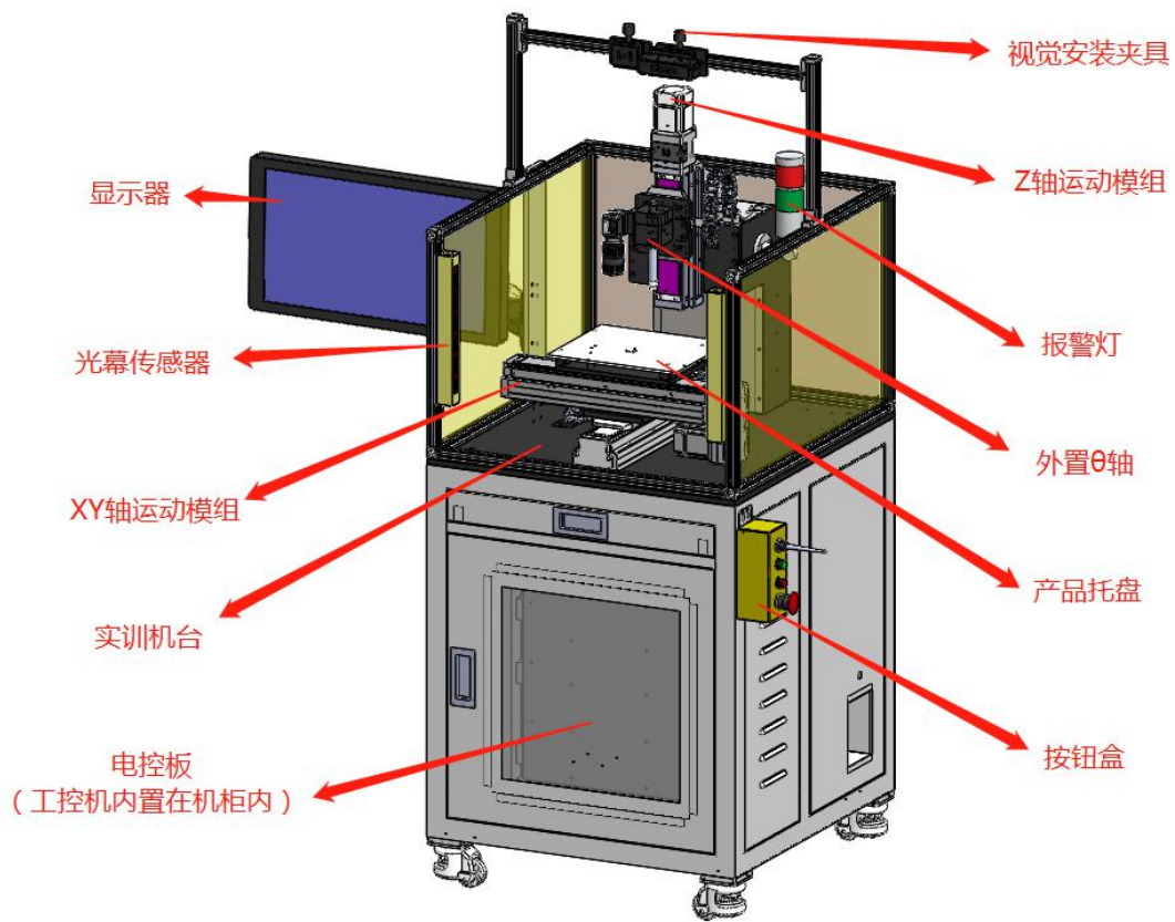
图4 设备组成图
