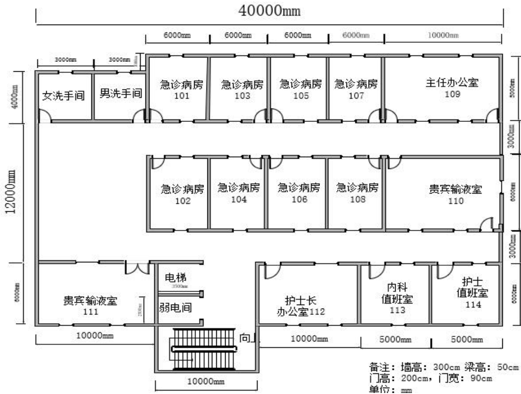
图 1 平面布局图
