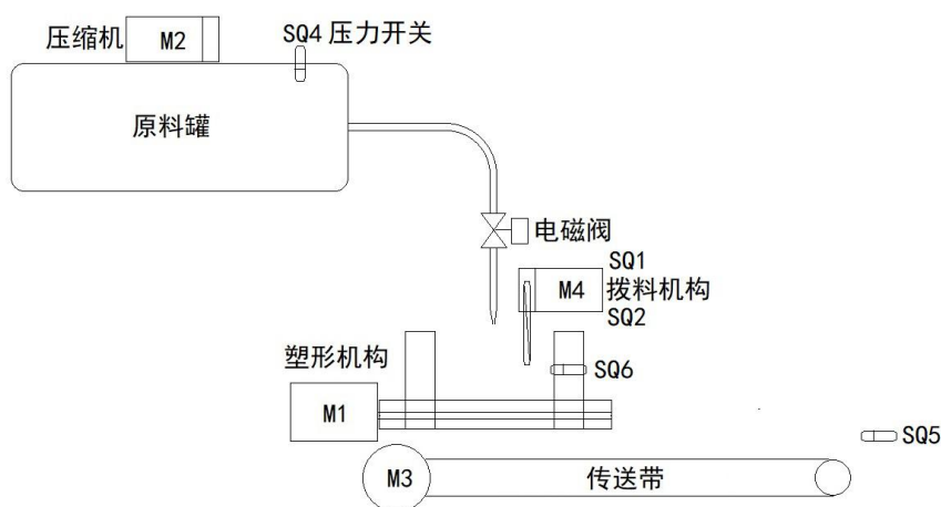
图 1 系统示意图
