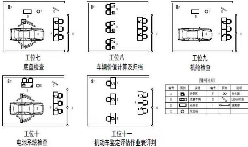
图5 机动车鉴定与评估作业模块场地布置图
