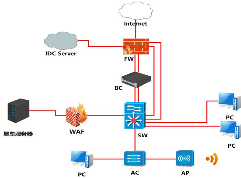
图 1 网络拓扑图
