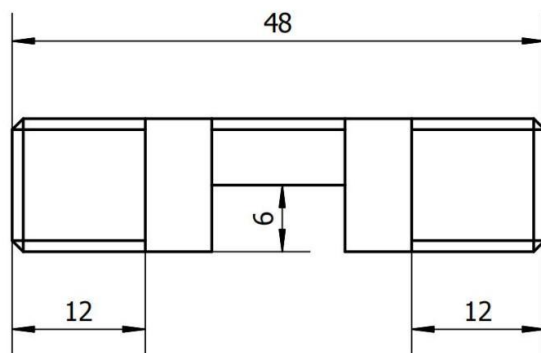
零件图：006
