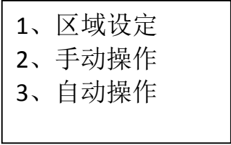
图 5 主界面
