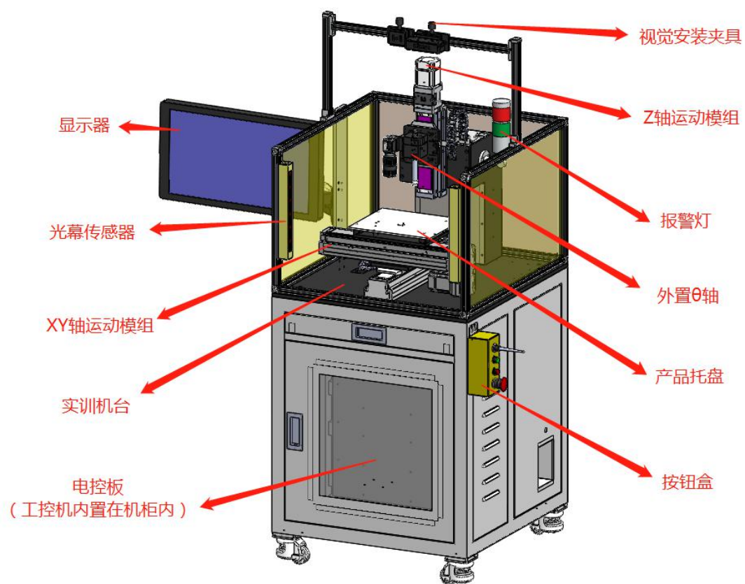
图 4 设备组成图
