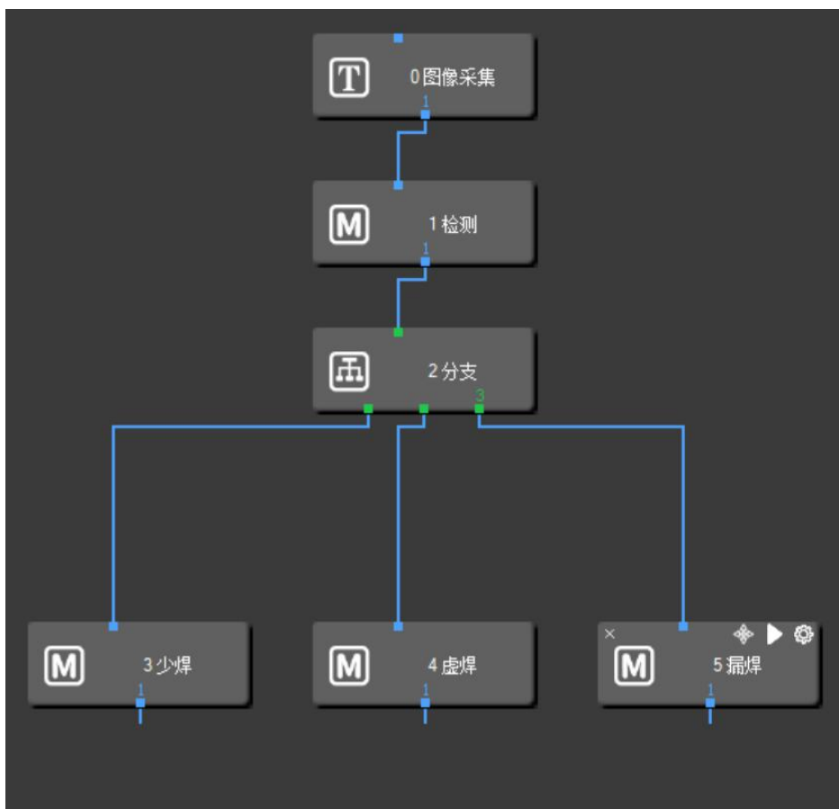
图 1 流程示意图
