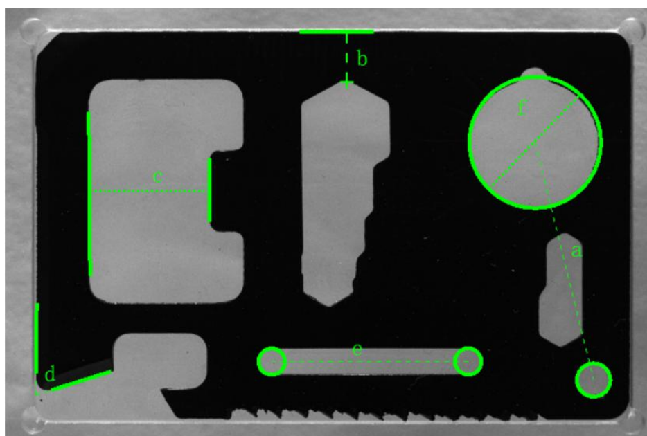
图 6 机械零件测量说明
