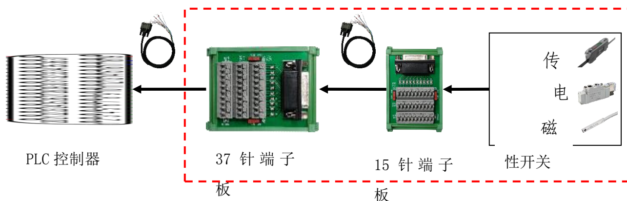
图B-2端子板连接示意图
