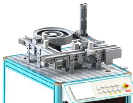
颗粒上料单元
