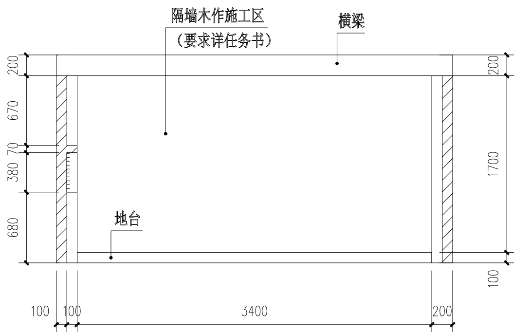
图6 C立面图
