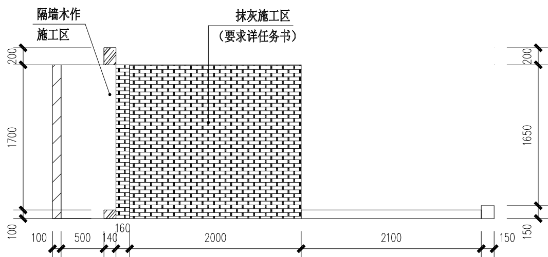
图5 B立面图
