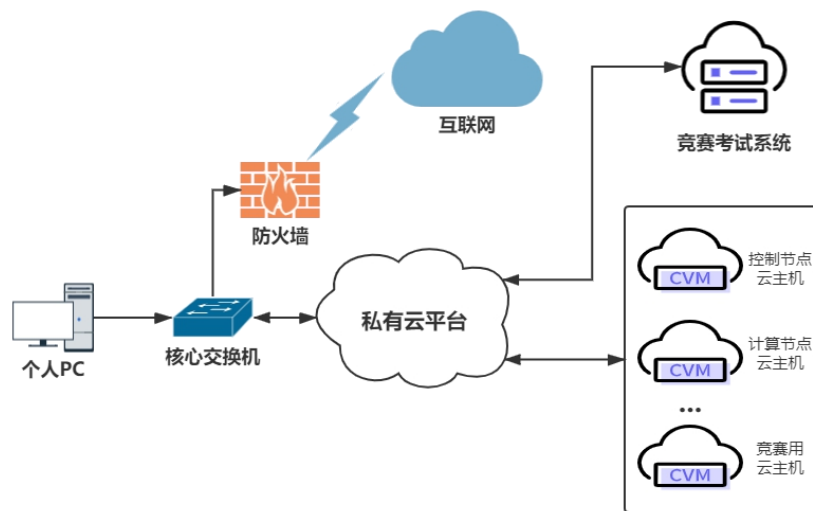
图 1 赛项系统架构图
