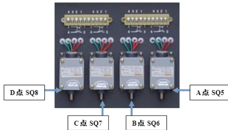
图 4 模拟传感器各检测点元件
