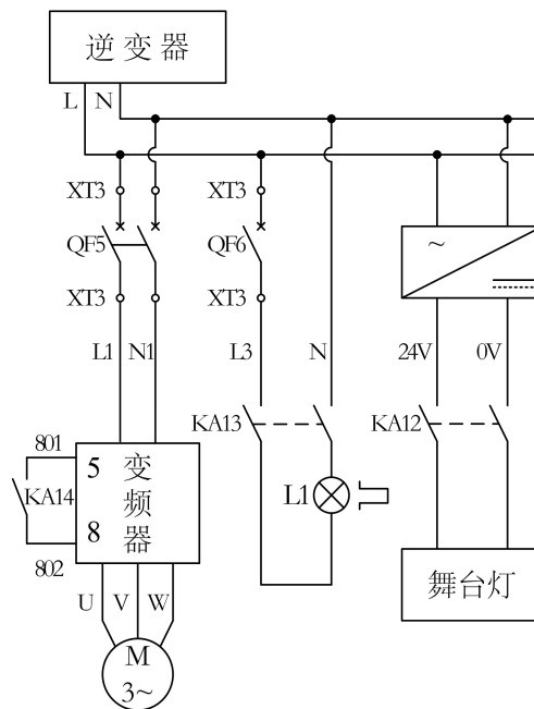
图 15 逆变与负载系统接线图
