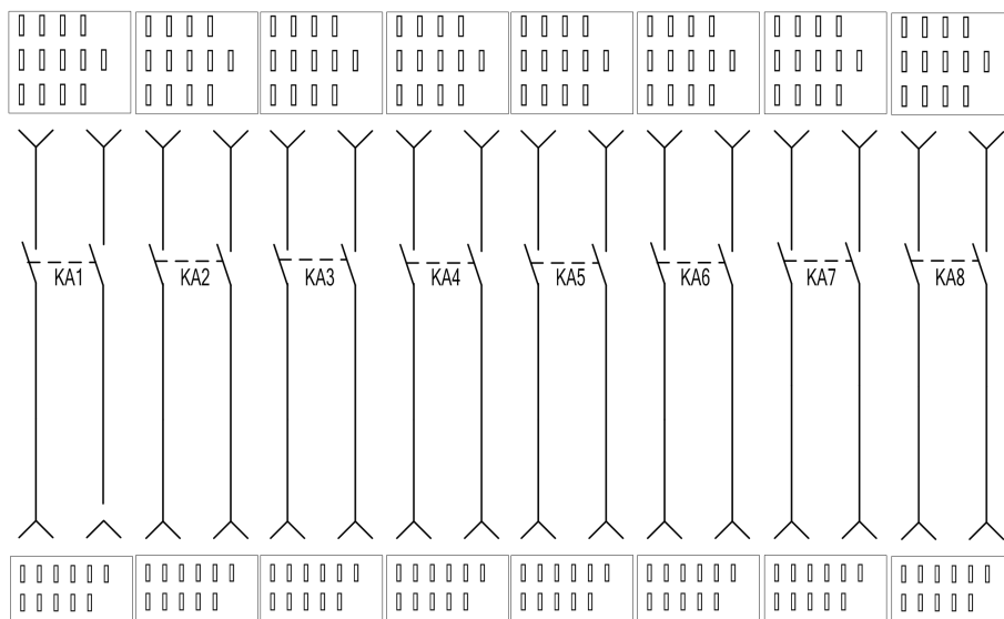
图 12 光伏供电系统继电器控制电路接线图二
