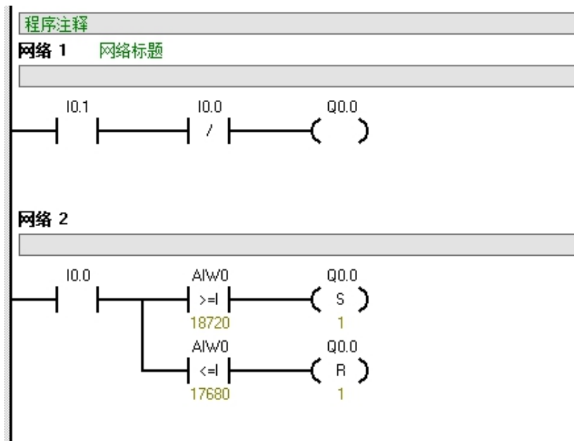
图 4.1 PLC 梯形图
