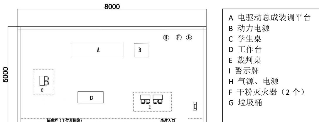
图 5 总成竞赛工位布置图
