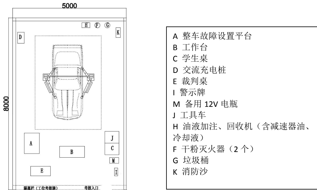
图 3 整车竞赛工位布置图 (“新能源汽车故障诊断与排除”和“新能源汽车维护与高压组件更换”模块)
